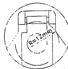
DETAHE 1 DISTÂNCIA MINIMAL PARA A OPERAÇÃO DE INSTALAÇÃO OU DE RETIRADA DO PARAFUSO DE SEGURANÇA COM O USO DA CHAVE MAGNÉTICA
