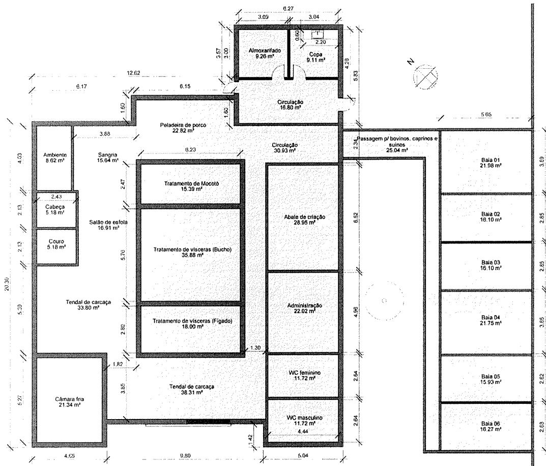
1 01 PLANTA BAIXA 1 : 120
