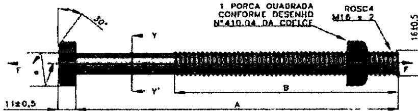
VISTA LATERAL
