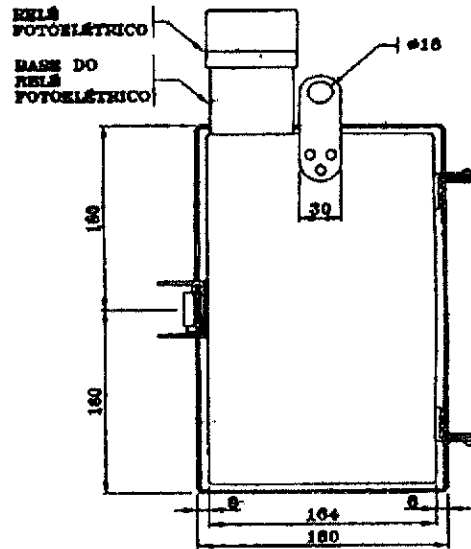
VISTA POSTERIOR
