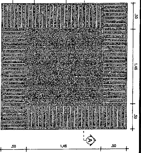
VISTA SUPERIOR BANCO/CANTEIRO 2,46 X 2,46 M
