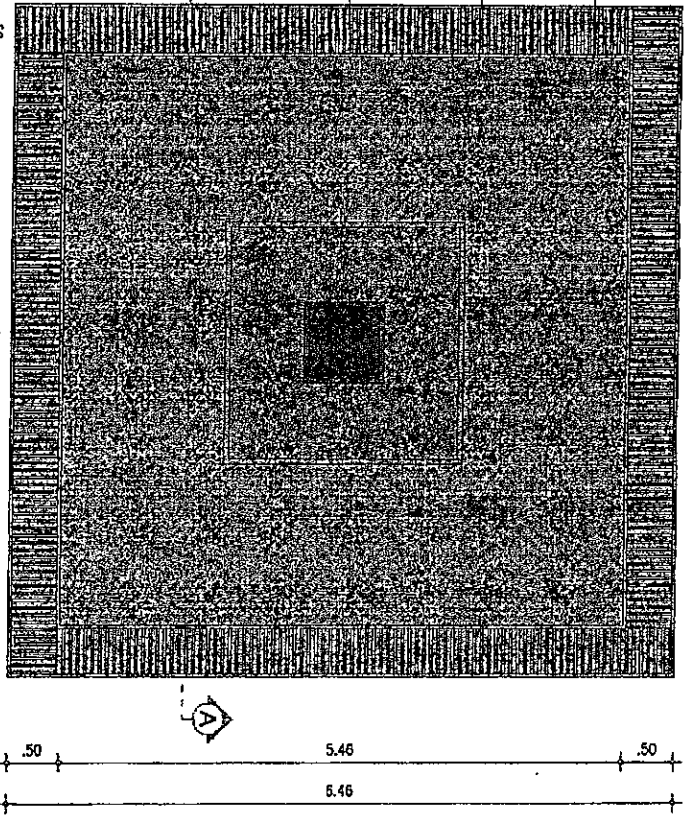
VISTA SUPERIOR BANCO/CANTEIRO 6,46 X 6,46 M
